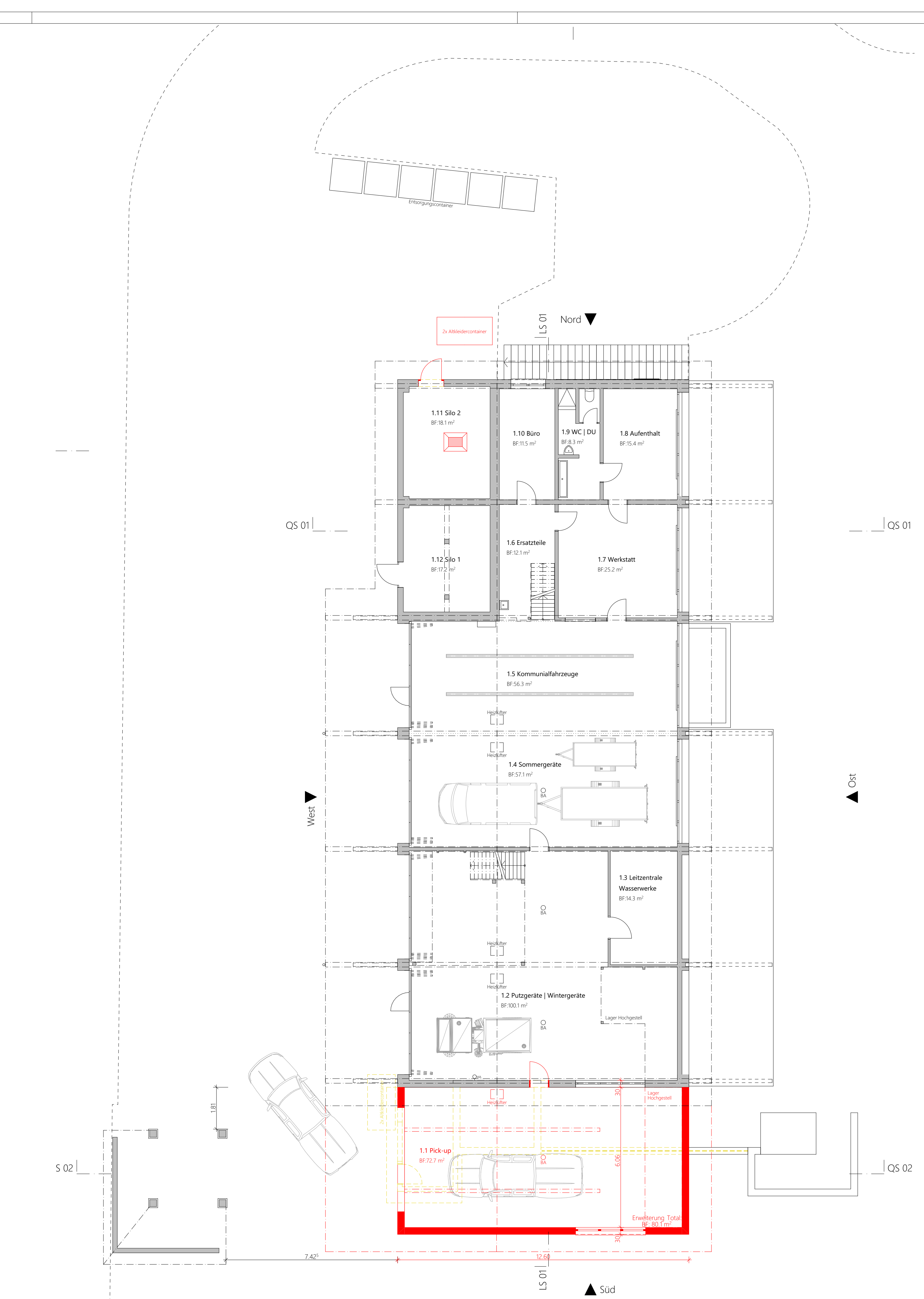
Obergeschoss Werkhof
