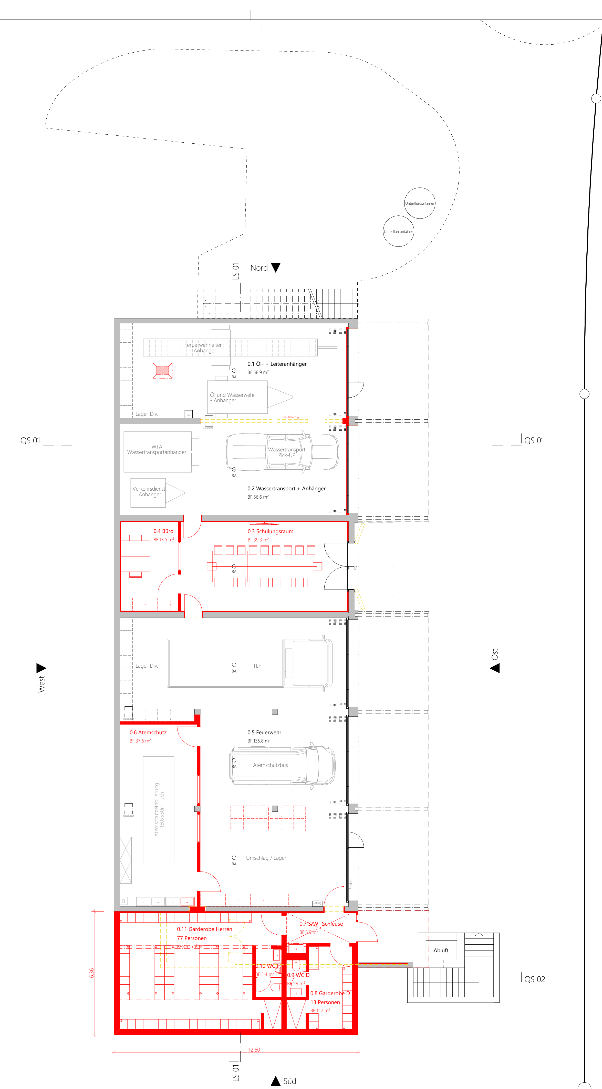
Erdgeschoss Feuerwehr
